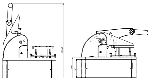
LHS2-Sonderhöhe 80mm
